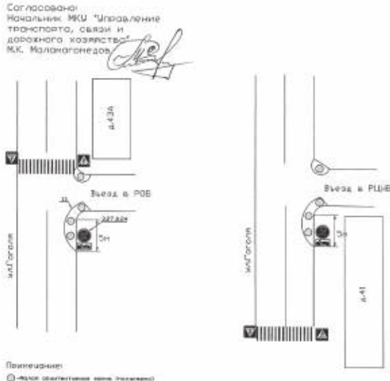
Схема организации дорожного движения по ул. Гоголя
